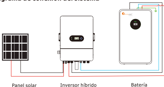
Figura 3-1 Diagrama de conexión del sistema con una sola batería
